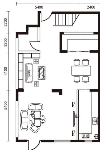
复式一层
